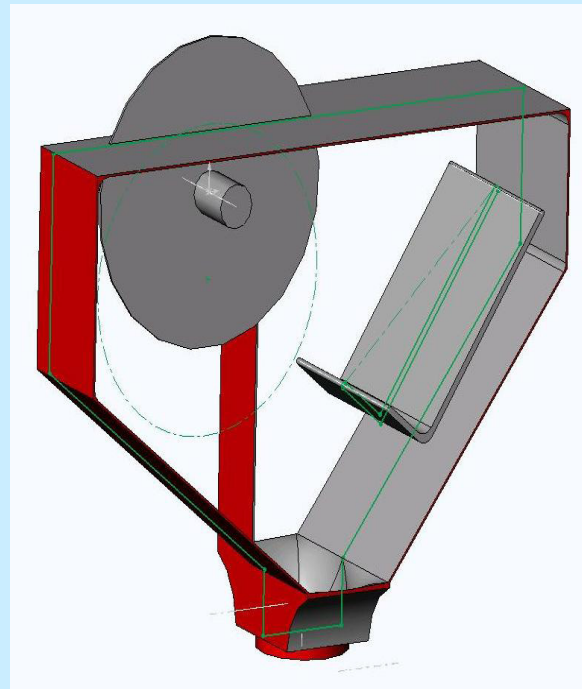
2. Spänefang
